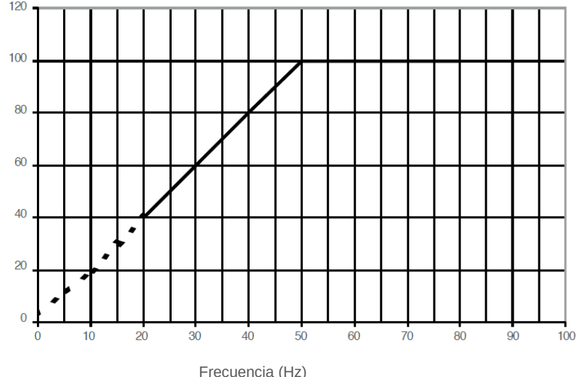
Tensión entrada en función de la nominal
